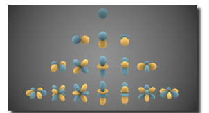
Harmoniques sphériques
